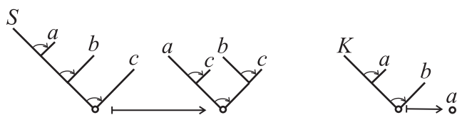
Рис. 1. Характеристики комбинаторов S и K .
